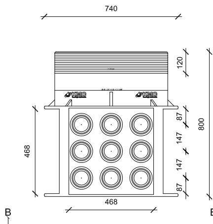
VIEW A-A
